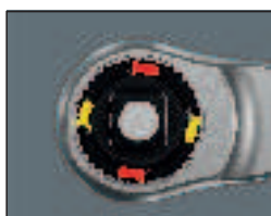
Uzębienie dwuzapadkowe, kąt wyzwalań max. 5°
